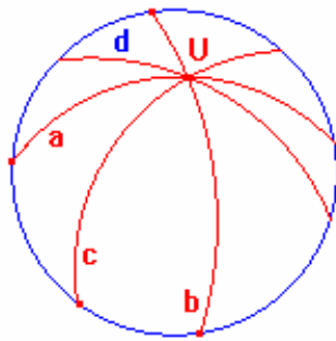
Figura 12a. a y b separan a c y d
