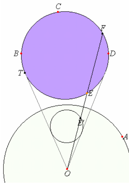
Figura 5. Inversión de un círculo.
