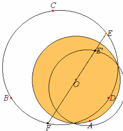
Figura 6. Inversión de un círculo con centro en el interior.
