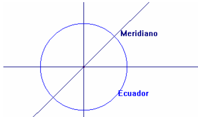
Figura 23. Representación de “rectas” en el plano estereográfico.
