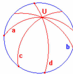
Figura 12b. a y b no separan a c y d .
