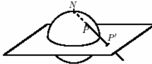
Figura 41. Proyección estereográfica en el plano \pi .
