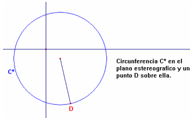
Figura 36. Representación en el plano estereográfico de la construcción 3.2.1.
