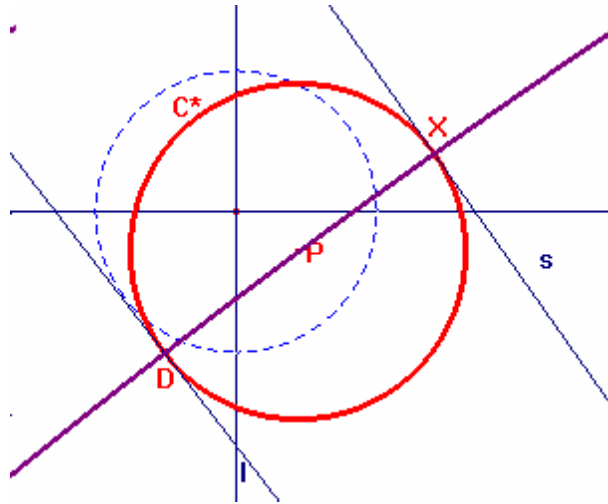
Figura 38. Perpendicular buscada cuando la recta es el ecuador.
