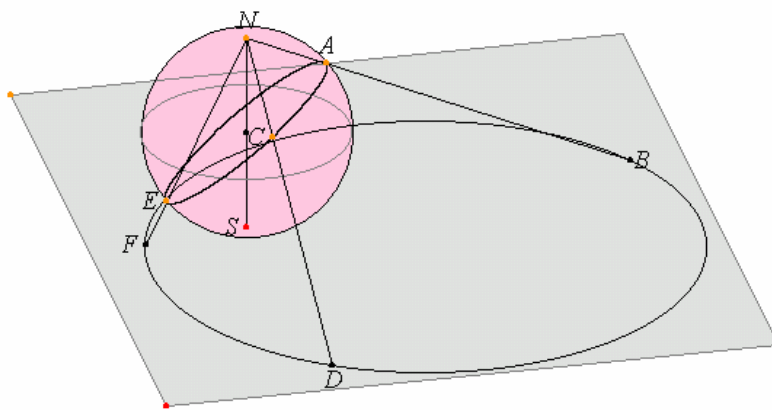
Figura 35. "Recta" en la esfera y un punto en ella.
